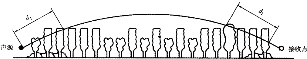
图 9 通过树和灌木时噪声衰减示意图
