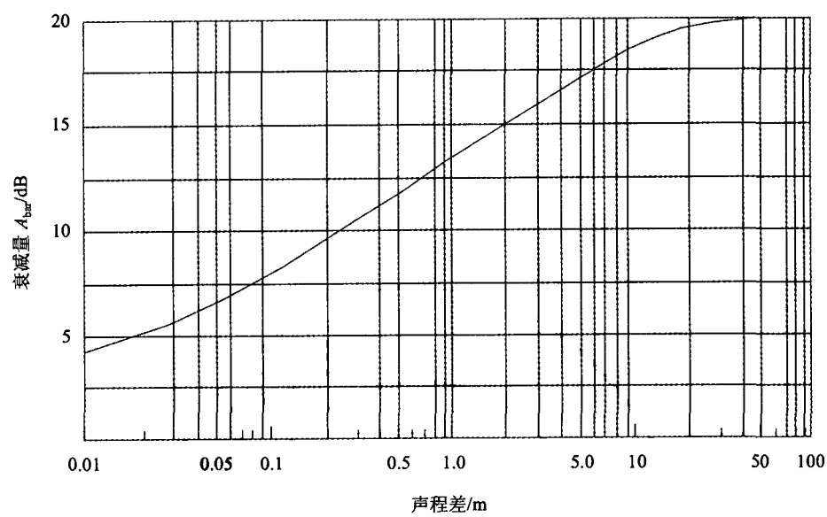
图 A.5 噪声衰减量 A_{\bar{a}} 与声程差 \delta 关系曲线 ( f=500\text{ Hz} )
