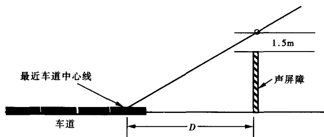
图 7 参考点位置 ( D > 15\text{m} )
