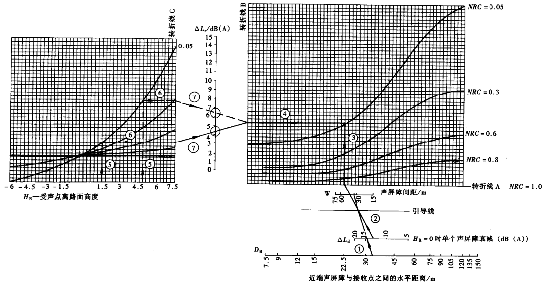
图 A.1 平行声屏障列线图的应用
